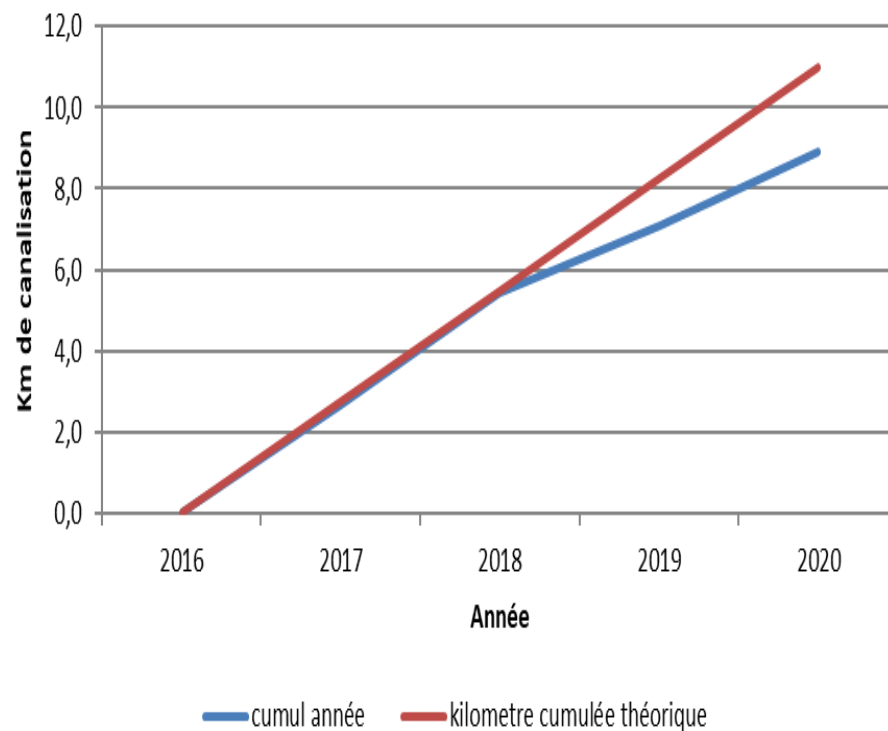
Suivi du curage préventif Castelmoron
