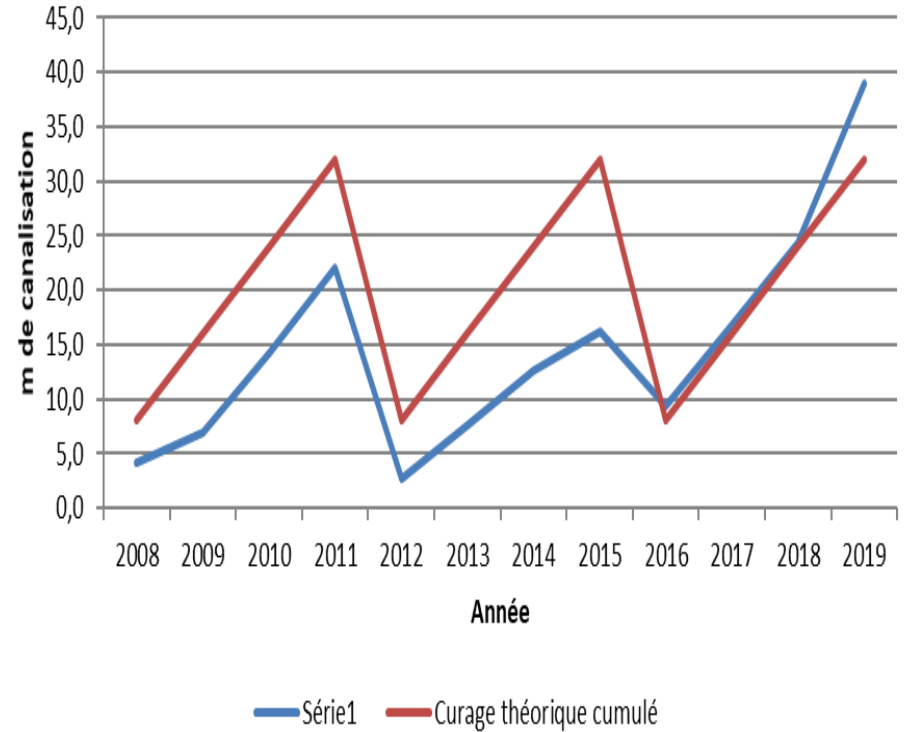
Suivi du curage préventif
