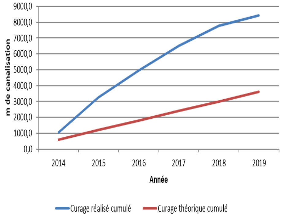
Suivi du curage préventif
